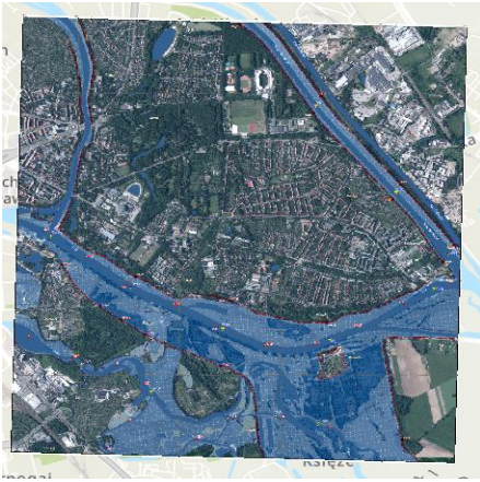
Prawdopodobieństwo wystąpienia powodzi 0,2% – raz na 500 lat
