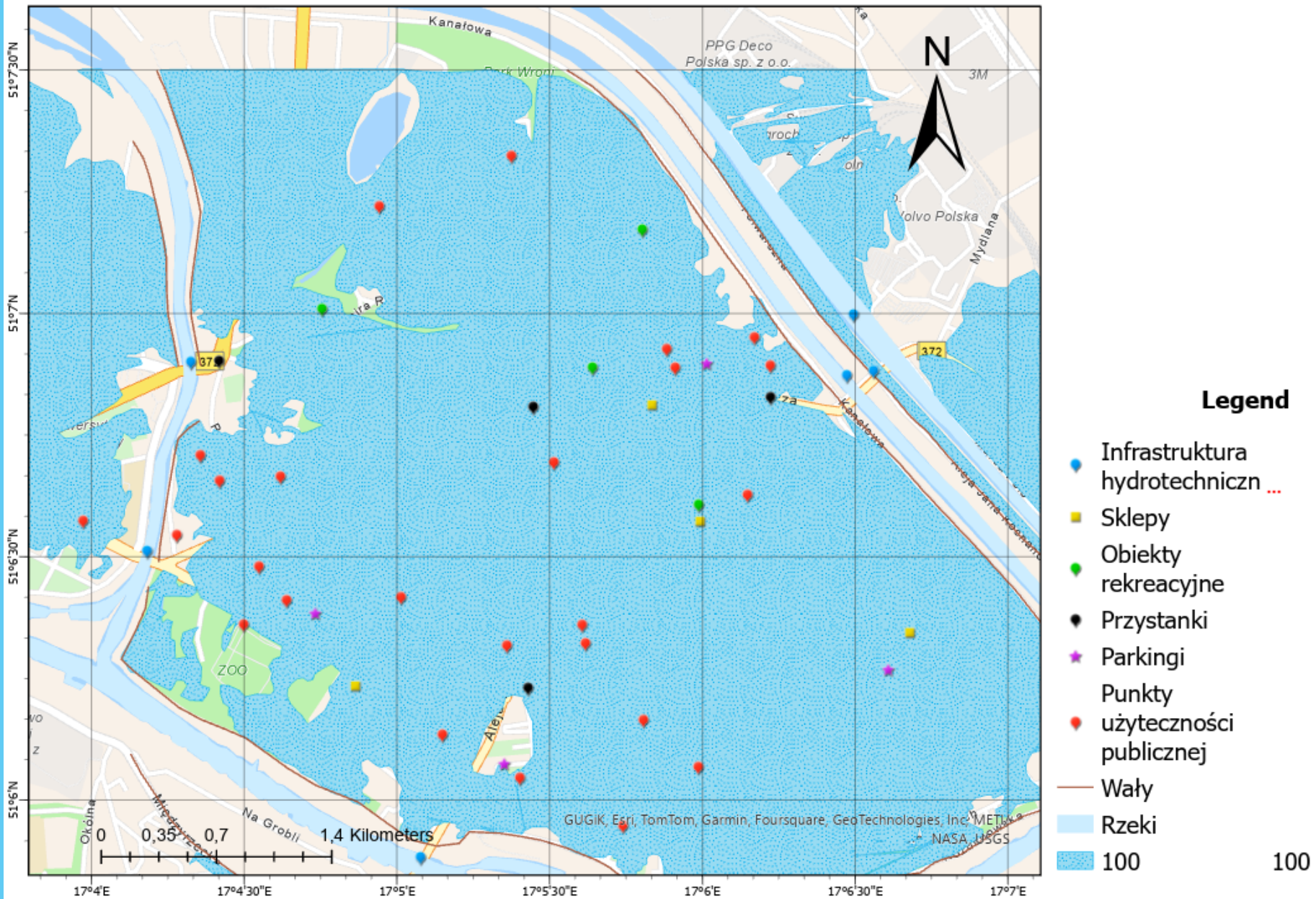
Mapa: Prawdopodobieństwo zagrożenia powodziowego z całkowitym pęknięciem wału
