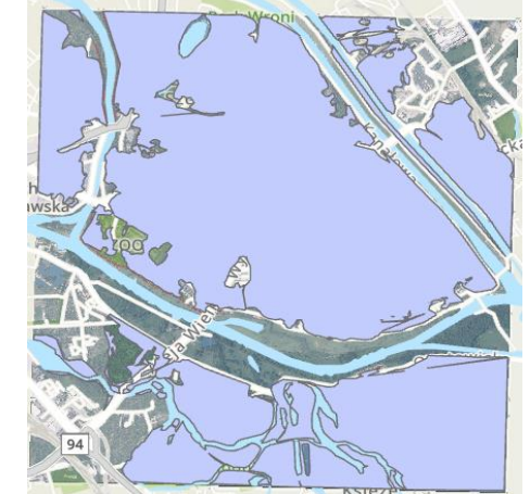
Scenariusz zniszczenia lub uszkodzenia wału przeciwpowodziowego
