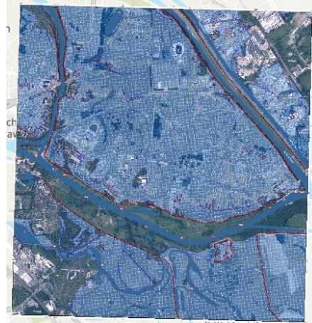
Scenariusz zniszczenia lub uszkodzenia wału przeciwpowodziowego
